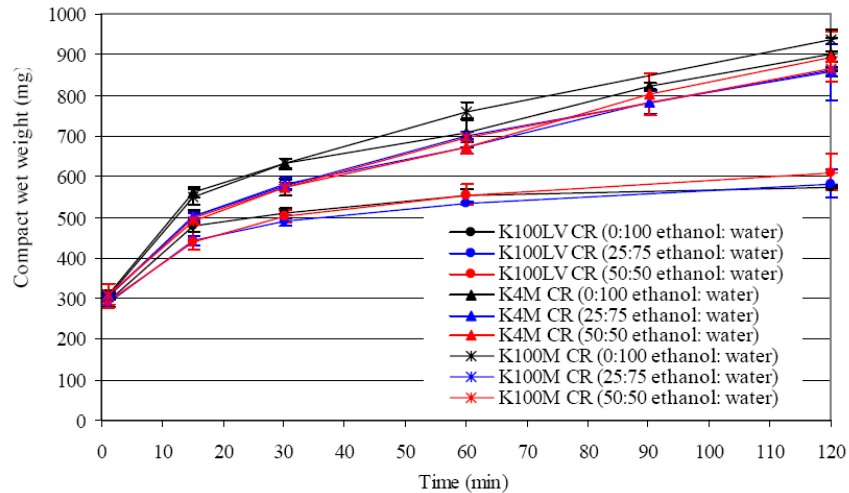
图1. 羟丙甲纤维素片剂的湿重
